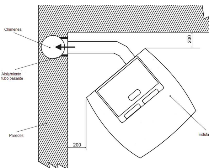
INSTALACIÓN EN ÁNGULO (mm)
